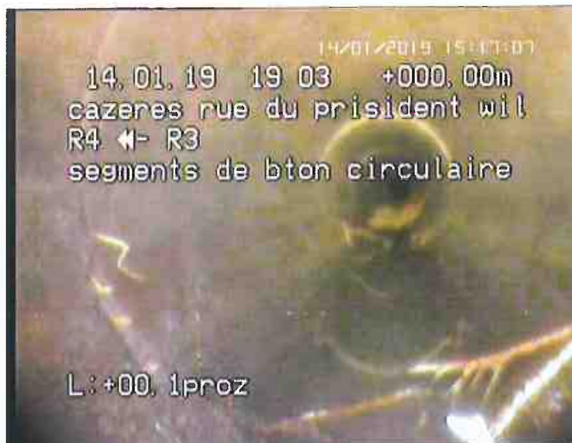
Photo: 5_5_71_A.jpg, N° support: 2-14012018 c_7, 00:00:02 0m, Noeud de départ, regard de visite R4
