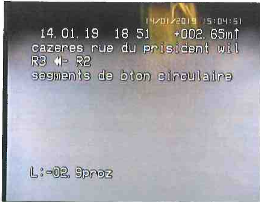
Photo: 4_4_70_A.jpg, N° support: 2-14012018 c_7, 00:00:35 2,65m, Ensemble complexe de racines de 3 à 9 h. réduction de la section transversale: 10 %
