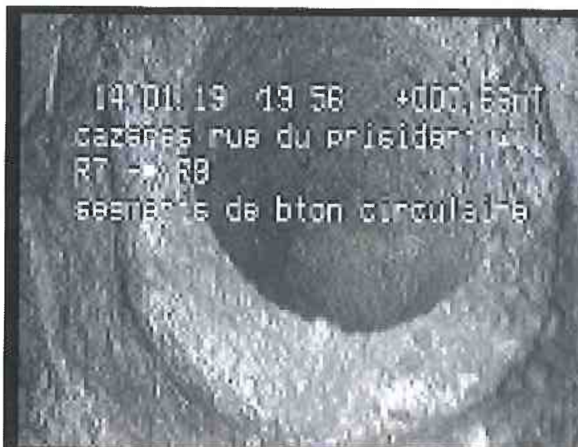
Photo: 9_9_39_A.JPG, N° support: 2-14012018 c_7 0,66m, Selle, carottée, raccordement ouvert à 10 h., hauteur: 100 mm, (largeur: 100 mm)
