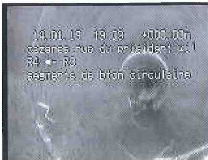
Photo: 5_5_9_A.JPG, N° support: 2-14012018 c_7 1,64m, Radicelles à 5 h. réduction de la section transversale: 5 %
