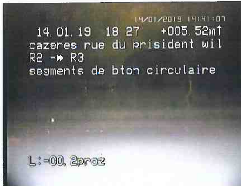
Photo: 3_3_68_A.jpg, N° support: 2-14012018 c_7, 00:00:47 5,51m, Niveau d'eau, aspect discontinu niveau exprimé en pourcentage du diamètre: 20 %
